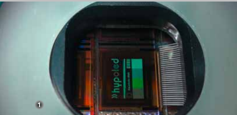
1 Test eines Mikrodisplays auf Waferlevel.
